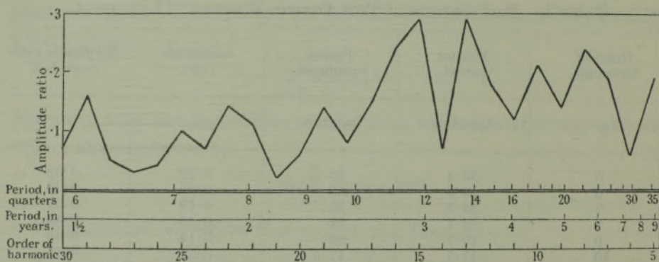
FIG. 2.—Periodogram.
